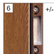
6 Dwie regulacje docisku rygli +/-
