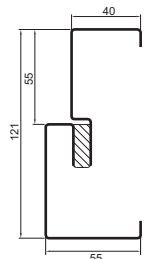
Ościeżnica stalowa NT/75
