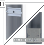
11 Elementy wzmacniające konstrukcję ościeżnicy z kółkami montażowymi lub bez 12. Ościeżnica 10/54,11/54 12. Ościeżnica 15/54
