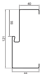
Ościeżnica stalowa S15/75
