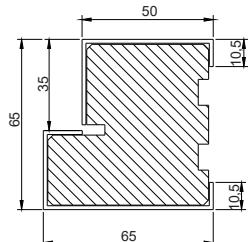
Ościeżnica drewniano-stalowa DS „L”/54
