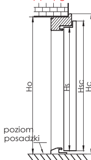
Drzwi trzy przyłgowe 3P
