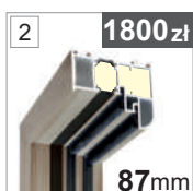
Ościeżnica aluminiowa ALU/90 trzykomorowa z podwójnym uszczelnieniem z przegrodą PCW wypełniona pianą
