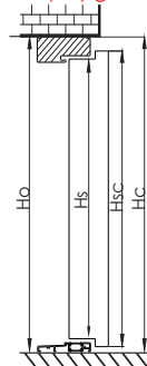
Drzwi cztero przyłgowe 4P
